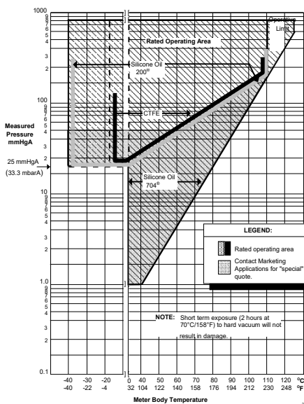
Рисунок 2. График зависимости давления от температуры сенсора STA822, STA82L
