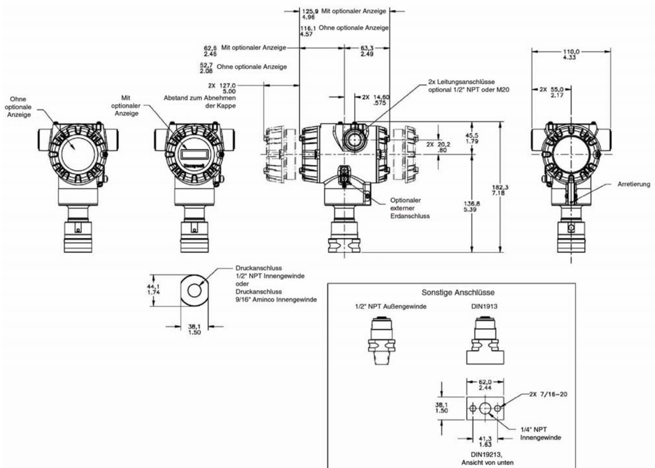
Abbildung 5 – Typische Montageabmessungen von STG84L, STG87L, STG88L und STG89L als Referenz
