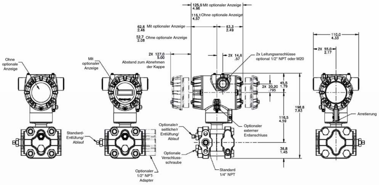
Abbildung 4 – Typische Montageabmessungen von STG840 und STG870 als Referenz
